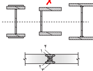
شکل ۴-۶ متعادل کردن جوش‌ها یا نوارهای جوش در حول تار خنثای عضو، اعوجاج زاویه‌ای را به صفر می‌رساند.
