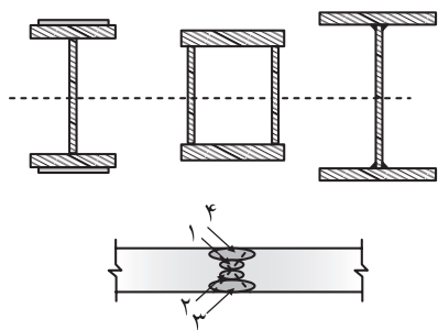
شکل ۴-۶ متعادل کردن جوش‌ها یا نوارهای جوش در حول تار خنثای عضو، اعوجاج زاویه‌ای را به صفر می‌رساند.
