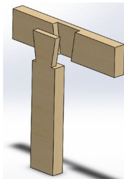
اتصال نیم و نیم وسط دم چلچله
