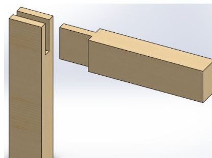
اتصال گوشه ای فاق و زبانه ساده
